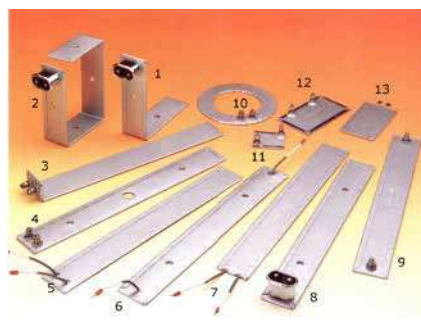
Resistencia-para-Selladora
